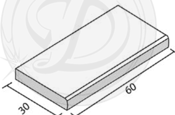
5-30-60 2 CANTOS BISELADOS
